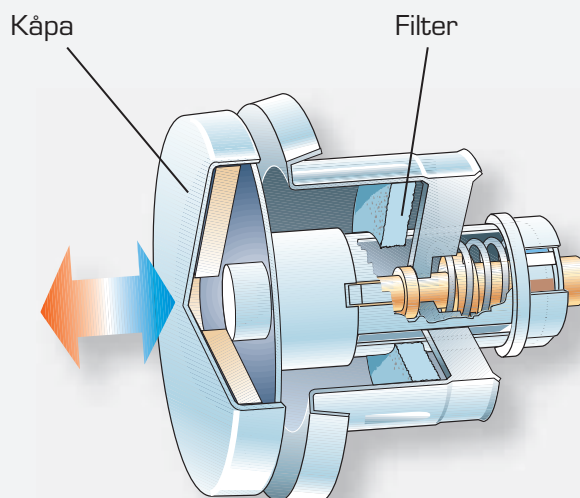
Fresh 100 Thermo-dB med 300 mm genomföring.
